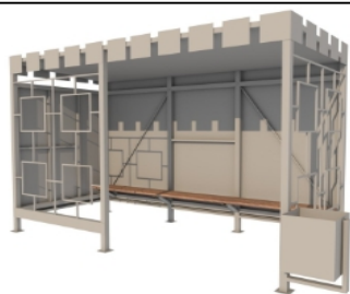
Остановочный павильон - ЛОТ №11 Габаритные размеры (ДхШхВ): 3500х1800х2400мм.
